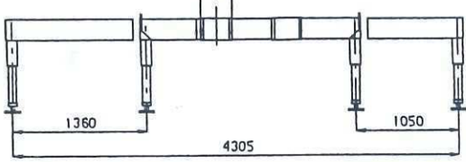
VERSIONE CON PIEDI TELESCOPICI
